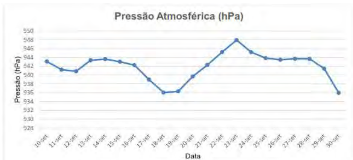
Gráfico 4 - Pressão Atmosférica de 10 a 30 setembro - ano 2019
