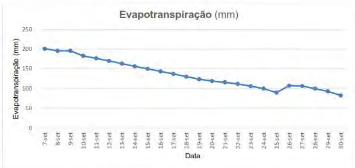
Gráfico 5 - Evapotranspiração de 07 a 30 setembro - ano 2019
