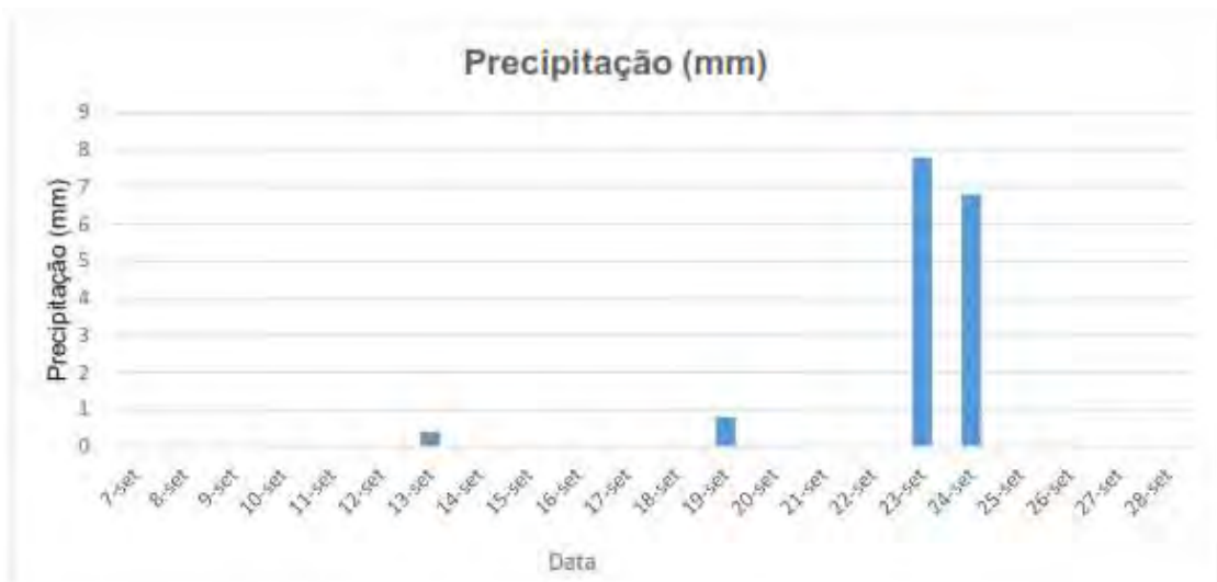
Gráfico 2 - Precipitação de 07 a 30 setembro - ano 2019
