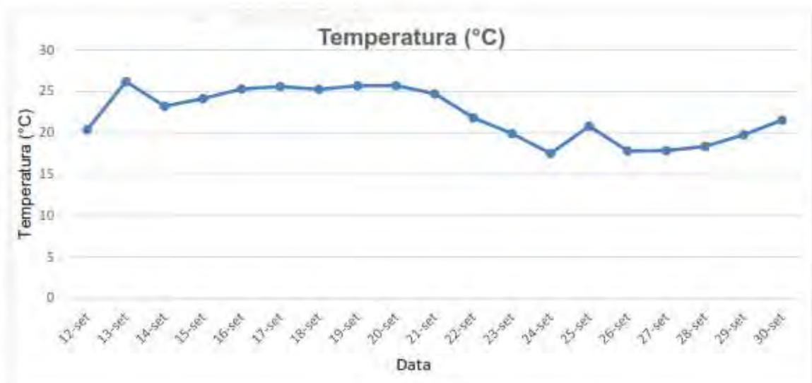
Gráfico 1 - Temperatura de 12 a 30 setembro - ano 2019
